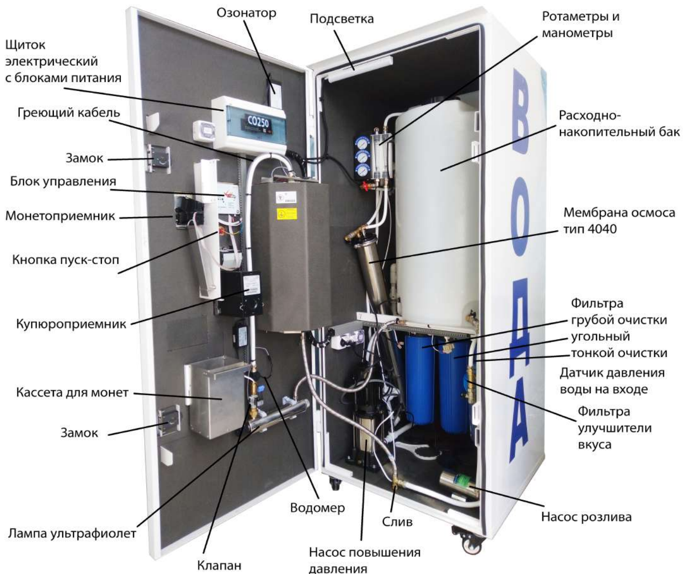
Рис3 Общий вид установки .
